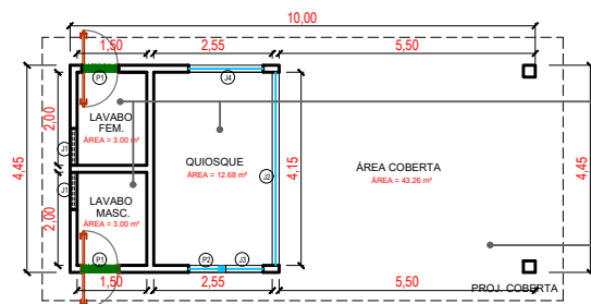
PLANTA BAIXA | QUIOSQUE ESCALA 1/125
