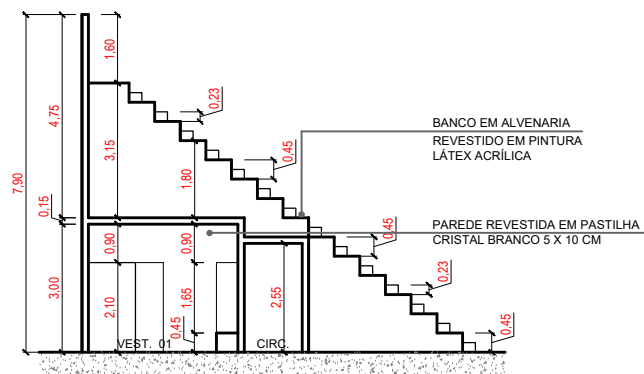
CORTE AA ESCALA 1/125
