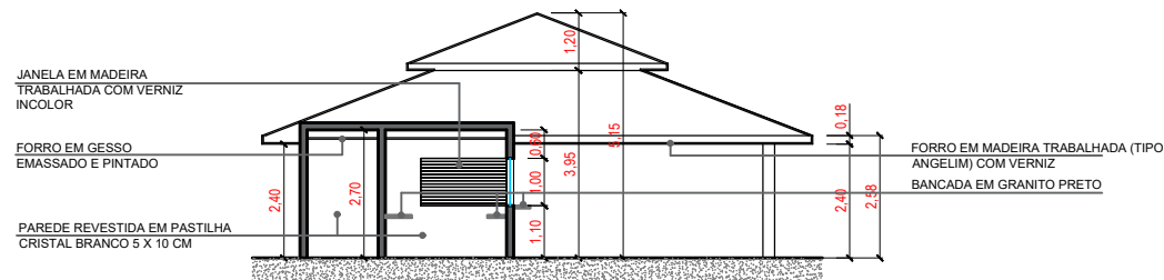
CORTE FF ESCALA 1/125
