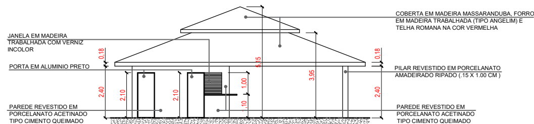
ELEVAÇÃO LATERAL ESCALA 1/125
