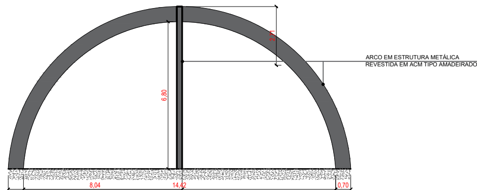
ELEVAÇÃO FRONTAL ESCALA 1/125
