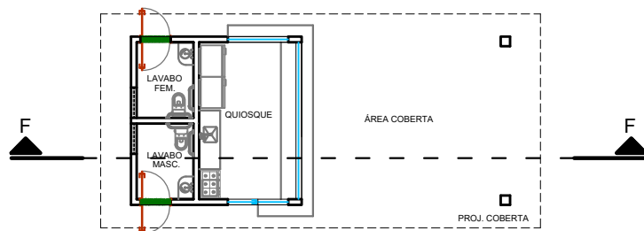
PLANTA BAIXA | LAYOUT | QUIOSQUE ESCALA 1/125
